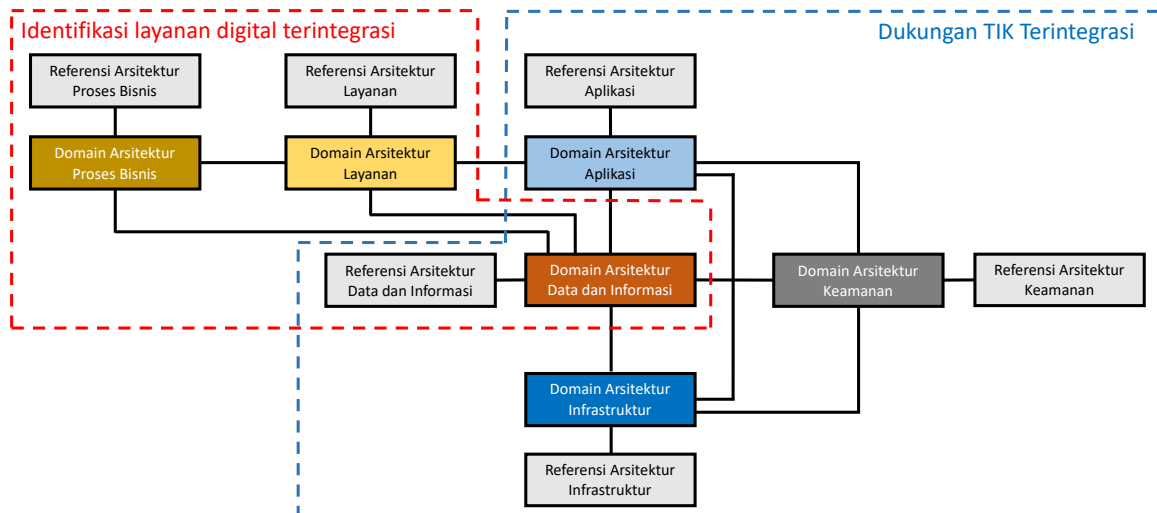
Gambar 8. Keterkaitan antar domain dan referensi pada arsitektur SPBE
