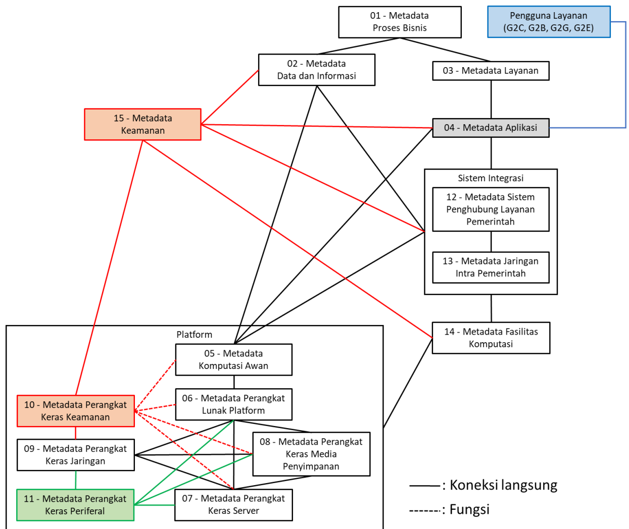
Gambar 9. Relasi Metadata Arsitektur SPBE
